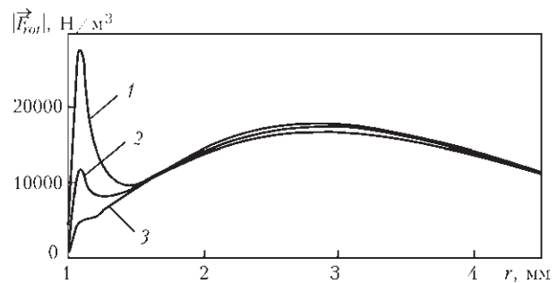
Рис. 14. Распределения вихревой составляющей силы Лоренца на поверхности анода при T_s = 500 \text{ K} : 1 — Q^0 = 1500 ; 2 — 500 Вт; 3 — обычная дуга
