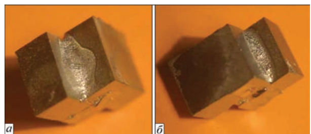
Рис. 3. Внешний вид нахлесточного соединения, паянного припоем №1: а — прямая галтель; б — обратная
