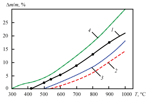
Рис. 10. Удельное увеличение массы порошков при нагреве на воздухе: 1 — \text{Fe}_3\text{Al} ; 2 — \text{Fe}_3\text{Al}(\text{Cr}, \text{Zr}) ; 3 — \text{Fe}_3\text{Al}(\text{Mg}) ; 4 — (\text{Fe}, \text{Ti})_3\text{Al}
