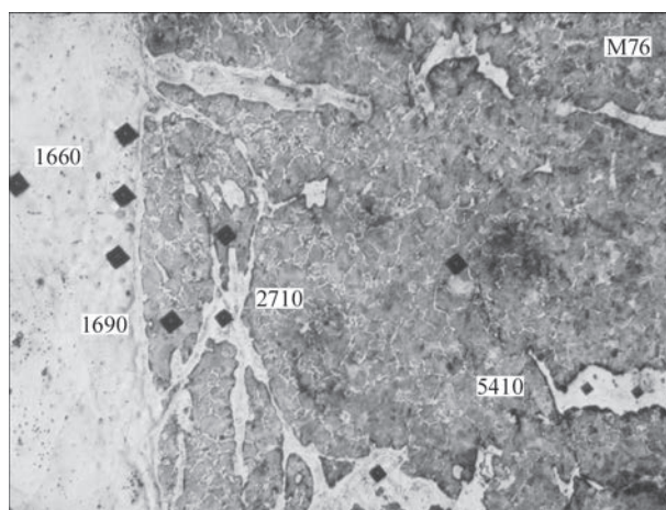
Рис. 7. Микроструктура ( \times 400 ) и распределение микротвердости в соединении рельсовой стали М76 и стали Гадфильда после отжига по режиму: T = 850 \text{ }^\circ\text{C} , \tau = 3 \text{ ч.} , охлаждение в масле
