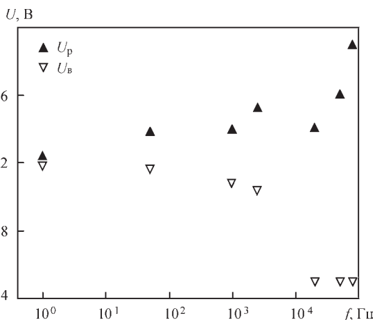
Рис. 14. Зависимости напряжения на дуге в импульсе ( U_p ) и в паузе ( U_b ) от частоты модуляции тока [15]
