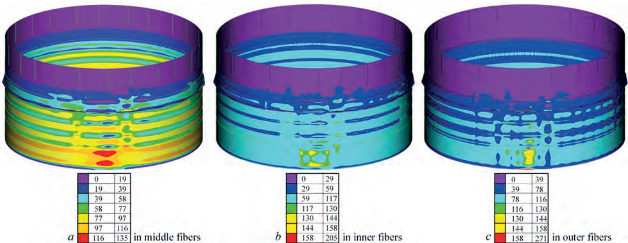
Fig. 4. Equivalent (von Mises) stress \sigma_{eq} , MPa in shell with rectangular depression formed after repair welding Рис. 4. Еквівалентні напруження по Мізесу \sigma_{eq} , МПа, в стінці з прямокутною недосконалістю, що утворилася після ремонтного зварювання
