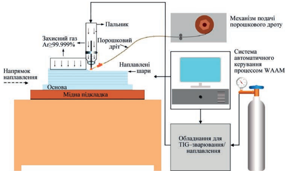
Рис. 3. Схема установки для послойного наплавления TIG способом с присадным металопорошковым дротом
