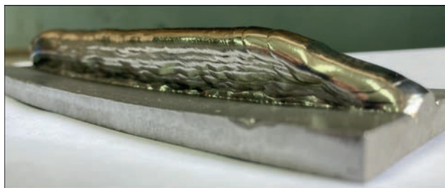
Рис. 8. Загальний вигляд дев'ятишарового зразка після процесу наплавлення присадним металопорошковим дротом на основі титанового сплаву системи Ti–Zr–Nb
