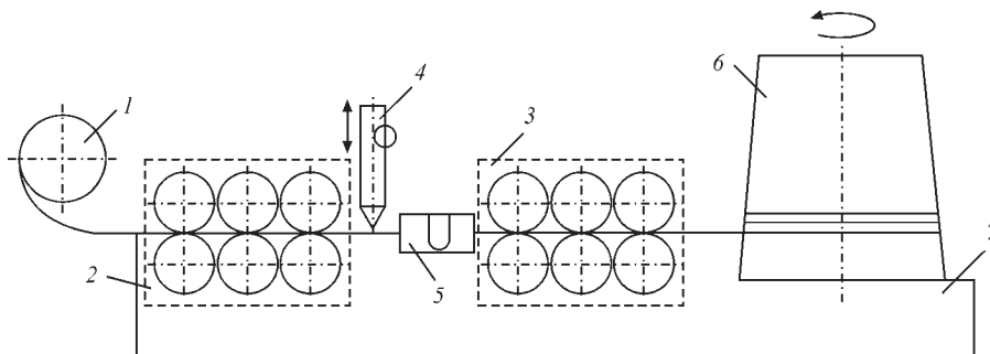
Рис. 1. Схема волочильного верстата для виробництва порошкового титанового дроту: 1 – касета; 2, 3 – роликові кліти; 4 – дозатор; 5 – U-подібна планка; 6 – барабан; 7 – станина
