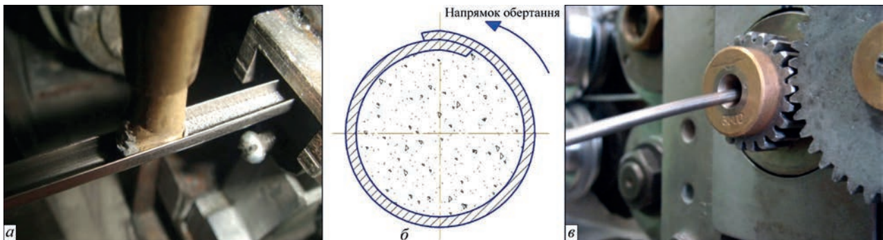
Рис. 2. Процес формування та перетяжки металопорошкового дроту: а – дозування шихти; б – схема закриття оболонки; в – філь'єра, що обертається
