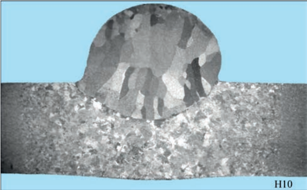
Рис. 4. Макрошліф отриманого трьохшарового зразка із застосуванням присадного порошкового дроту на основі титанового сплаву BT22
