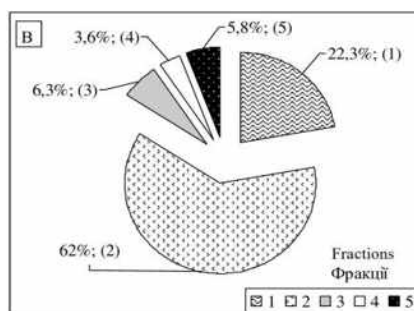
Схил ІІІ берми автомобільного відвалу Першотравневого кар'єру ПрАТ «ПівніГЗК»
