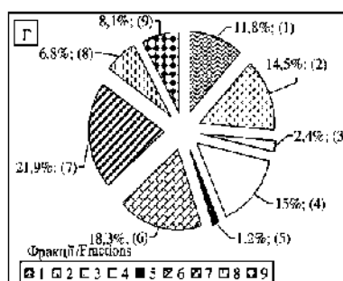
Схил ІІІ берми автомобільного відвалу Першотравневого кар'єру ПрАТ «ПівніГЗК»
