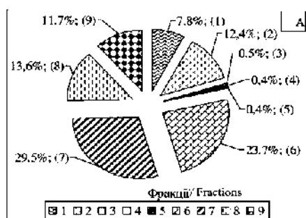
Схил ІІ берми автомобільного відвалу Першотравневого кар'єру ПрАТ «ПівніГЗК»
