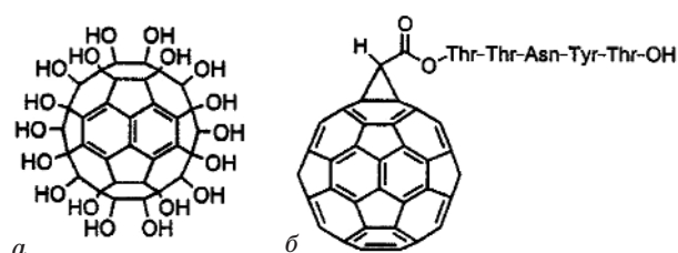
Рис. 3. Водорозчинні похідні фулеренів C_{60}
