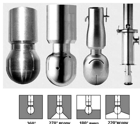
Головки, що обертаються, серії Toftejorg SaniMidget
