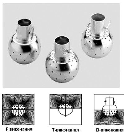
Нерухомі кульові головки LKRK
