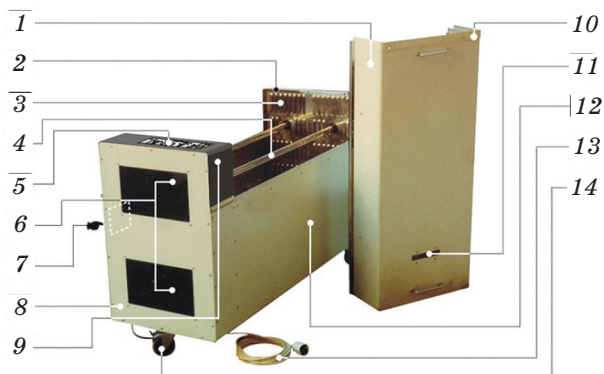
Рис. 16. Установка УФОЗОН 2099 (НВФ «Медведица», Росія):
