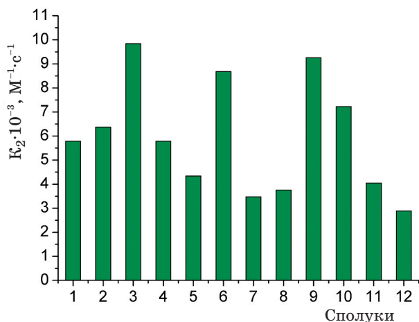
Рис. 2. Діаграма констант швидкості реакції для синтезованих похідних тіазолу з ДФПГ
