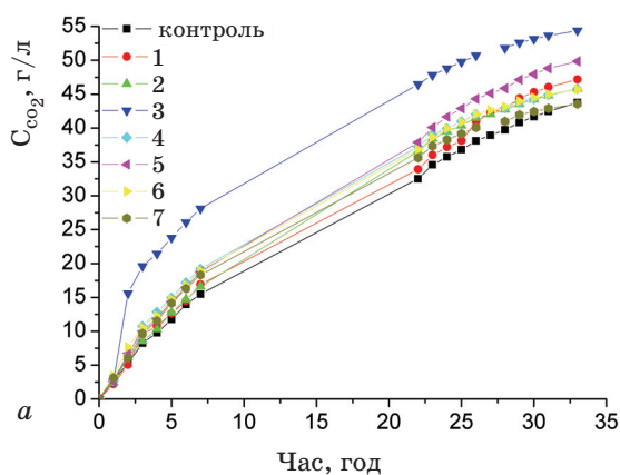
Рис. 3. Кінетичні криві виділення \text{CO}_2 дріжджовими клітинами в присутності синтезованих похідних тіазолу
