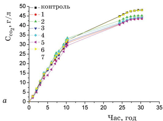
Рис. 5. Кінетичні криві виділення вуглекислого газу суспензією дріжджових клітин у присутності синтезованих похідних тіазолу, закріплених на поверхні кремнезему
