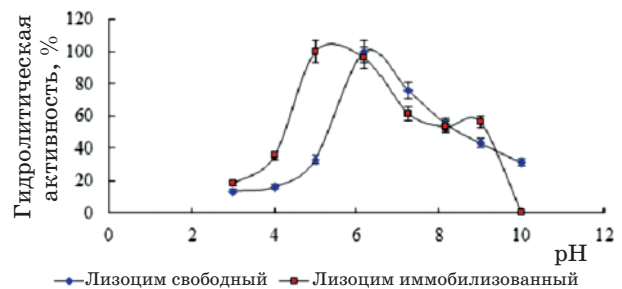
Рис. 2. Зависимость гидролитической активности свободного и иммобилизованного лизоцима от pH инкубационной среды ( M \pm m , n = 5 )
