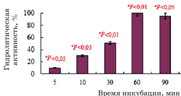
Рис. 4. Динамика высвобождения лизоцима из пленки (рН 6,2, 37 °С)
