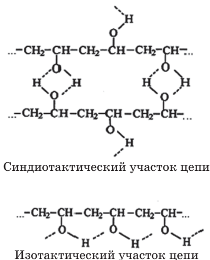
Рис. 1. Структура криогеля поливинилового спирта [6]
