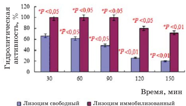
Рис. 3. Зависимость гидролитической активности свободного и иммобилизованного лизоцима от времени инкубации (рН 5,5, n = 5 )
