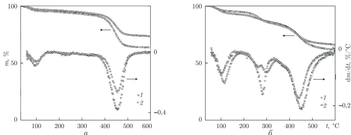
Рис. 2. ТГА термограммы образцов на основе \text{SiO}_2 -ПВП (а) и \text{SiO}_2 -ПАК (б): исходный гибриды (1) и AgНЧ-содержащий нанокompозит (2)
