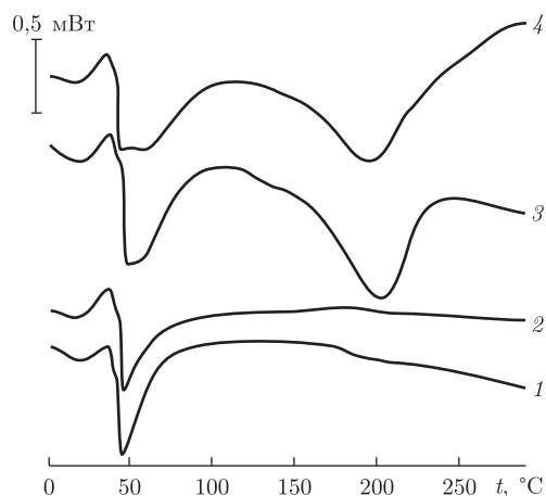
Рис. 3. ТМДСК термограммы общего теплового потока \text{SiO}_2 -ПВП (1), \text{SiO}_2 -ПВП/AgНЧ (2), \text{SiO}_2 -ПАК (3) и \text{SiO}_2 -ПАК/AgНЧ (4)
