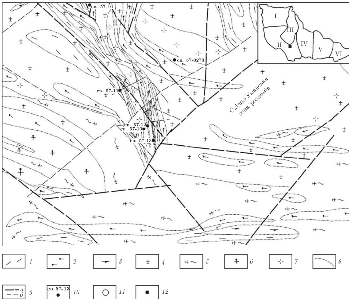
Рис. 1. Схематична геолого-структурна карта кристалічного щита центральної частини Гайворонського рудопроюву за матеріалами ПЗЕ-46 КП "Кіровогеологія".
