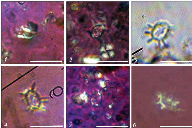
Рис. 2. Порівняння розміру коколітів роду Stephanolithion із келовейських відкладів різних розрізів (знімки виконані в єдиному масштабі): 1 – г. Веселий шпиль; 2 – с. Горбані; 3 – яр Маланчин потік; 4 – Мар'їн яр; 5 – св. Глухівська-319 (інтервал 297,2–300,9 м); 6 – Мар'їн яр
