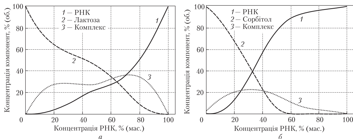
Рис. 2. Концентраційні профілі компонент, отримані за допомогою MCR-ALS аналізу для ІЧ спектрів, сумішей РНК–лактоза (а) та РНК–сорбітол (б)
