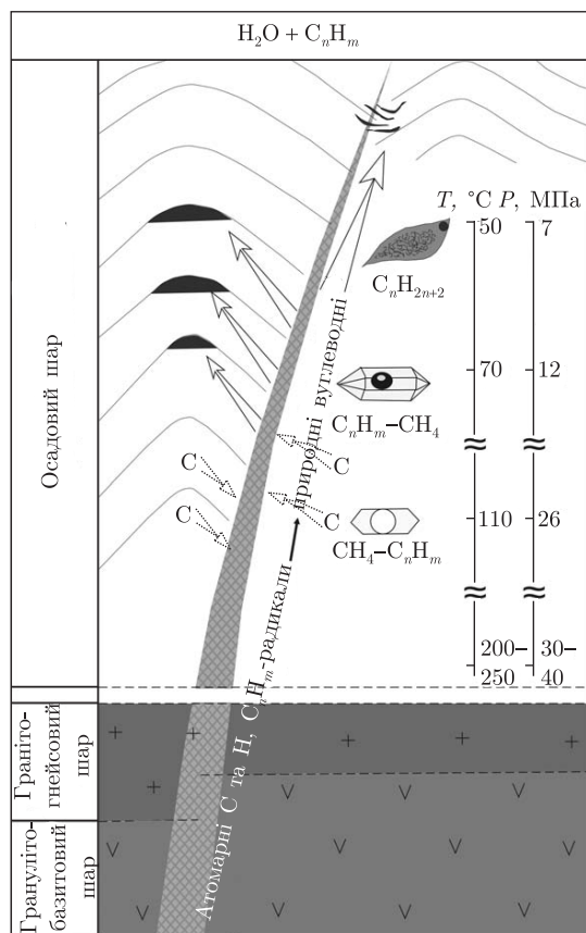
Рис. 2. Принципова схема міграційних процесів у флюїдопровідних розломних зонах підвищеної проникності гірських порід у вуглепородних масивах за участю вуглеводнів, синтезованих у середовищі глибинного високотемпературного флюїду (на прикладі жильних утворень Белз-Милятинської зони насувів у межах Львівського палеозойського прогину [15]) (на основі рисунка з праці [8] з деталізацією)
