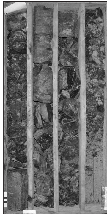
Рис. 2. Различная степень саморазрушения керна карбонатных пород уолсортских куполов в зависимости от глубины залегания.
