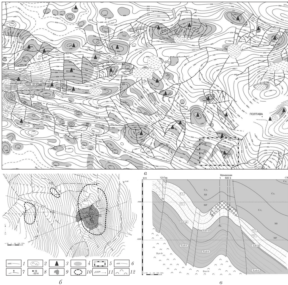
Рис. 4. Оценка нефтегазоносности уолортских куполов Днепровско-Донецкого региона: а — перспективы нефтегазоносности уолортских куполов центральной части ДДВ на глубинах более 5 км; б — установленная и предполагаемая нефтегазоносность разуплотненных уолортских куполов на Новодиканьско-Мачехском участке южного моноклиналичного склона приосевого грабена; в — геологический разрез по линии фрагмента регионального профиля Зачепиловка–Бельск.
