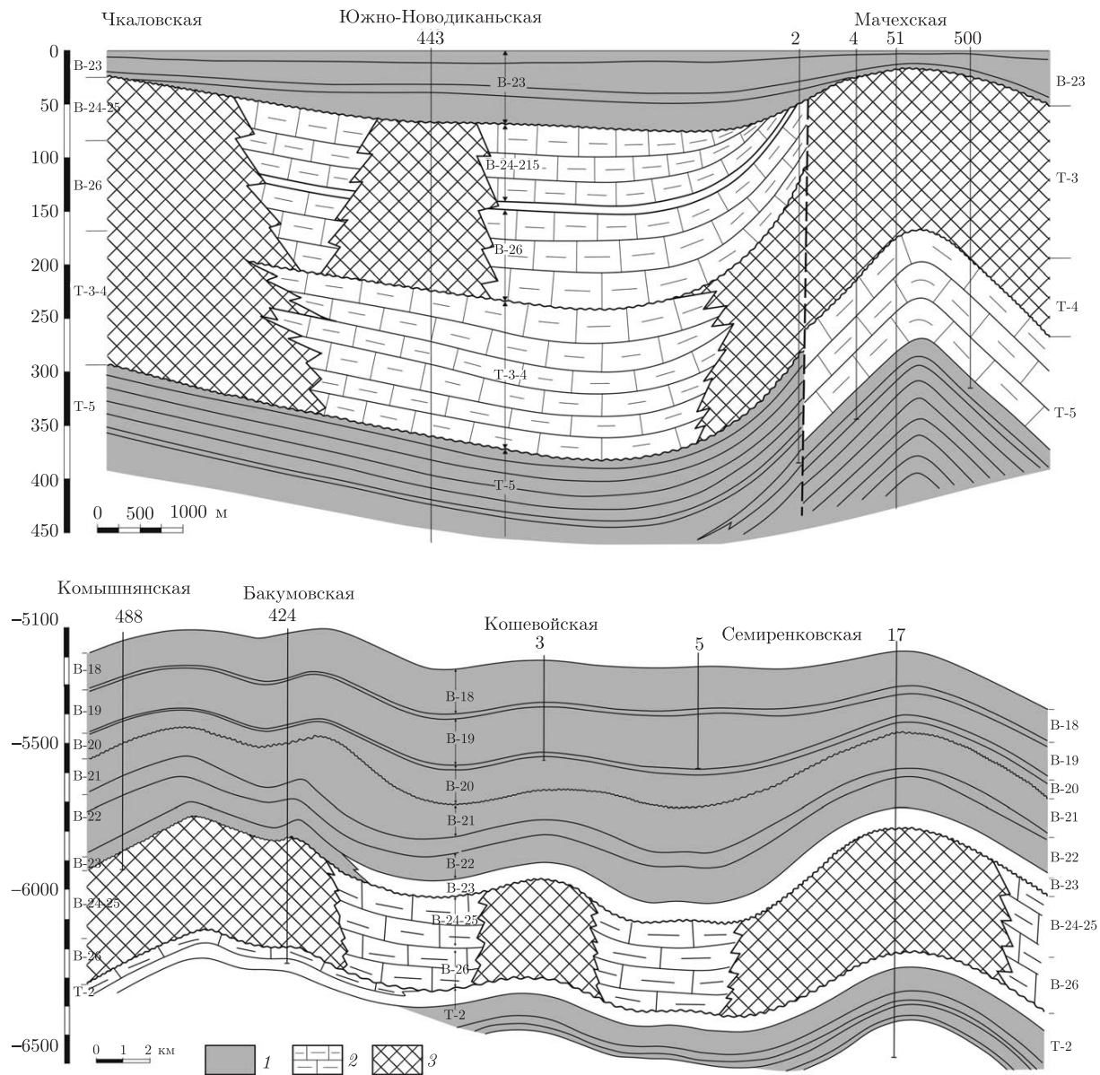
Рис. 3. Литолого-палеотектонические разрезы турнейско-нижневизейских отложений центральной части ДДВ.
