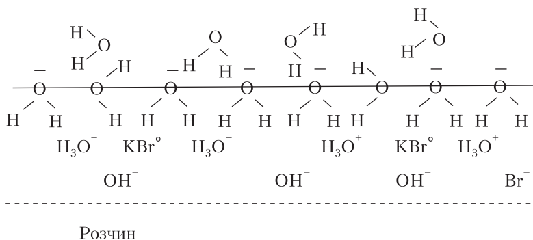
Рис. 2. Молекулярна схема будови інтерфейсу водного розчину KBr. Внаслідок самочинної орієнтації молекул H 2 O на поверхні виникає структурно обумовлений негативний заряд. У самому інтерфейсі під впливом поверхневого заряду формуються два шари іонів: шар з H 3 O + і шар з OH - . Сума всіх зарядів на одиницю площі негативна. Тому негативний і дзета-потенціал розчину [4]
