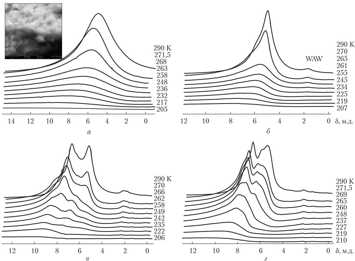
Рис. 3. Снятые при разных температурах спектры ^1\text{H} ЯМР композитной системы \text{SiO}_2 /хитозан 1/1 на воздухе ( a ), в среде \text{CDCl}_3 ( б ) и смеси 7/1 \text{CDCl}_3 /TFAA ( в , г )
