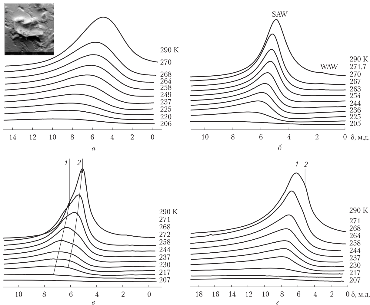
Рис. 1. Снятые при разных температурах ^1\text{H} ЯМР спектры хитозана, содержащего адсорбированную воду в воздушной среде (а), в среде \text{CDCl}_3 (б–з) с добавками трифторуксусной кислоты (ТФУК) (в, з) и \text{CD}_3\text{CN} (з)
