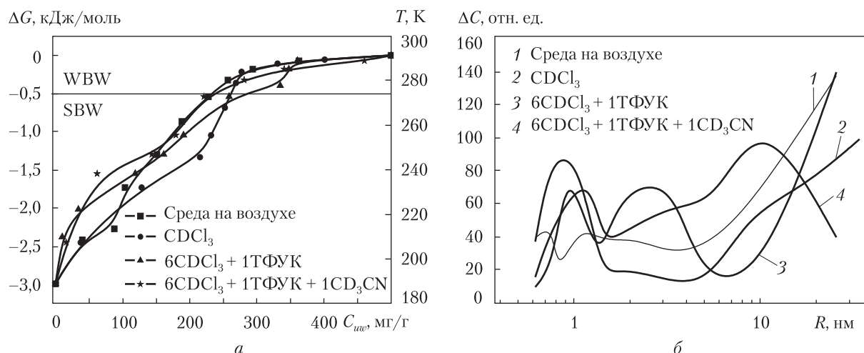
Рис. 2. Температурные зависимости концентрации незамерзающей воды и зависимости изменения свободной энергии Гиббса от концентрации незамерзающей воды (а); распределения по радиусам кластеров (доменов) адсорбированной воды (б) в гидратированном хитозане ( C_{H_2O} = 500 мг/г)
