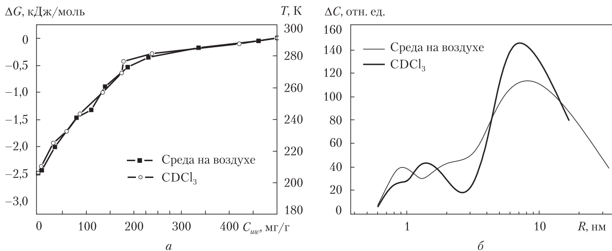
Рис. 4. Температурные зависимости концентрации незамерзающей воды и зависимости изменения свободной энергии Гиббса от концентрации незамерзающей воды ( а ); распределения по радиусам кластеров (доменов) адсорбированной воды ( б ) в гидратированном композите \text{SiO}_2/\text{хитозан} ( C_{\text{H}_2\text{O}} = 500 мг/г)
