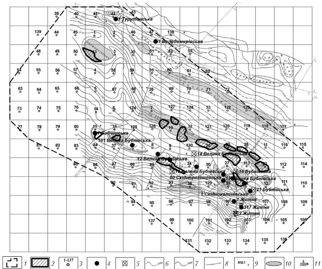
Рис. 1. Турутинсько-Рогінцівська зона структур. Структурна карта за горизонтами відбиття V_{B_{2п}} та V_{B_3} з результатами попередніх аерокосмічних досліджень. Умовні позначення: 1 – район дослідження; 2 – оптичні аномалії; 3 – номер спостережень; 4 – продуктивні свердловини; 5 – непродуктивні свердловини; 6 – ізогипси відбивного горизонту V_{B_{2п}} ; 7 – ізогипси відбивного горизонту V_{B_3} ; 8 – розривні порушення; 9 – свердловини глибокого буріння; 10 – перспективні об’єкти, що потребують подальшого вивчення; 11 – проектні свердловини
