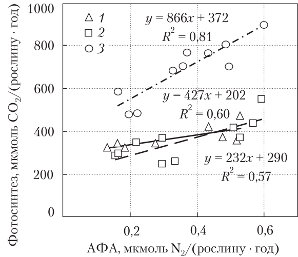
Рис. 1. Залежності між азотфіксувальною активністю та інтенсивністю фотосинтезу рослин сої, оброблених різними препаратами фунгіцидної дії в комбінації з лектином. Тут і на рис. 2, 3: 1 – фаза трьох справжніх листків; 2 – фаза бутонізації; 3 – фаза масового цвітіння
