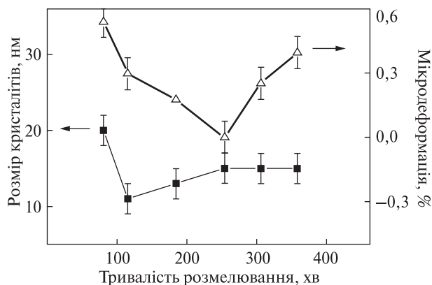
Рис. 4. Залежності розміру кристалітів та мікродеформації кристалічної ґратки карбіду \text{NiC}_x
