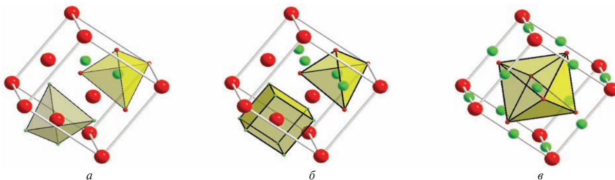
Рис. 3. Координаційні багатогранники атомів нікелю та вуглецю при описанні структури карбіду \text{NiC}_x в моделях структури типу \text{ZnS} (а) та \text{CaF}_2 (б), а також в структурі твердого розчину ( \text{Ni,C} ) (червоні кола – атоми нікелю, зелені кола – атоми вуглецю)
