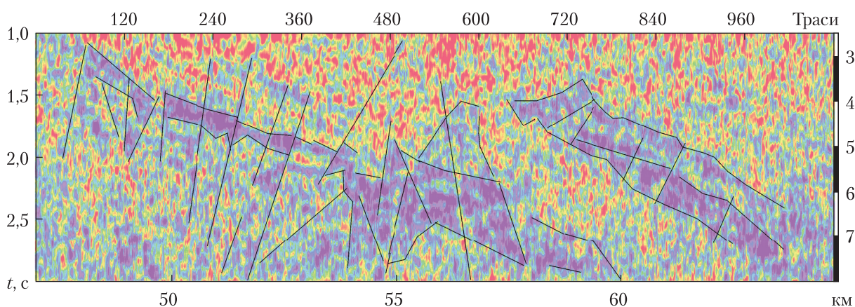
Рис. 4. Часові розрізи ЛДЗ з відміченими розломами, сформованими в покрівлі фундаменту
