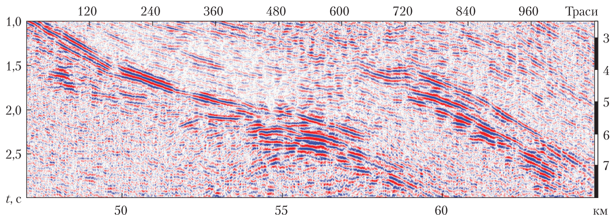
Рис. 1. Сейсмічне хвильове поле частини профілю DOBRefraction-2000, завдовжки 18 км з відображенням Ялинського насуву
