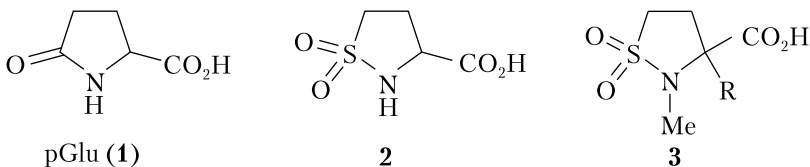
Рис. 1. Піроглутамінова кислота (1) та її сульфаізостери
