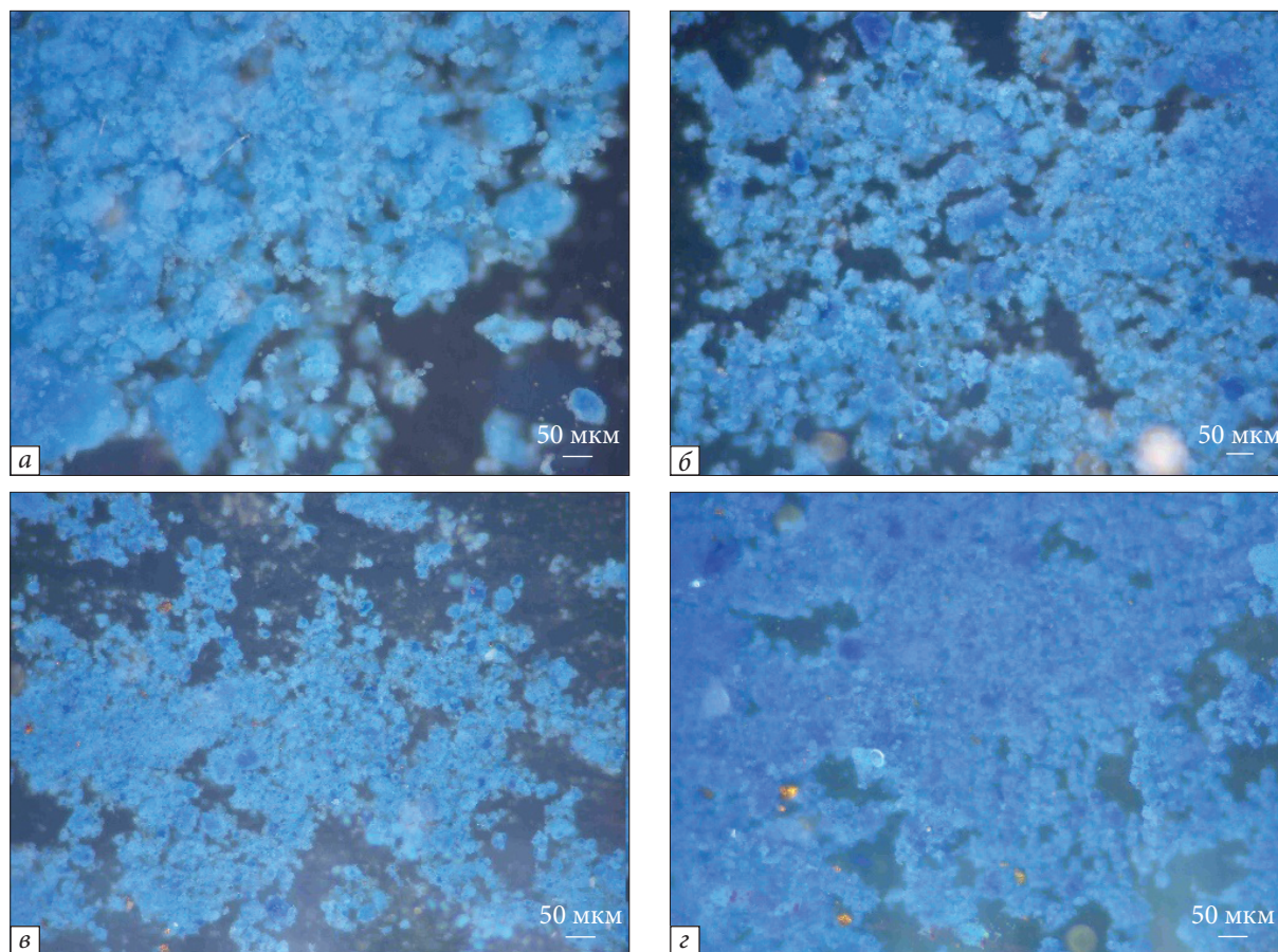
Рис. 2. Мікрофотографії композитів на основі А-300 з різним вмістом МС: а — 1 мас. %; б — 2 мас. %; в — 4 мас. %; г — 8 мас. % (відбиття, ×100)
