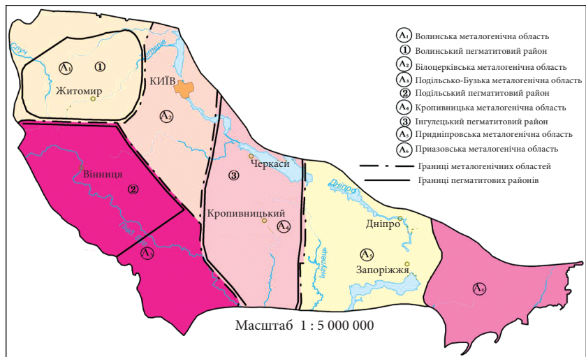
Рис. 9. Схема металогенічно-го районування Українського Щита
