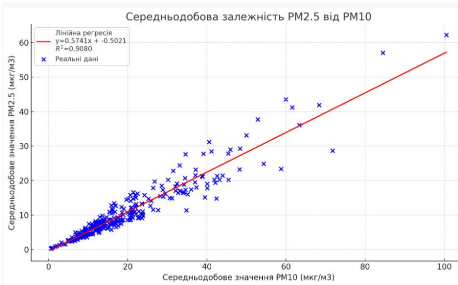
Рис. 5. Залежність середньодобових змін концентрацій частинок пилу PM2,5 та PM10 для території з антропогенним навантаженням
