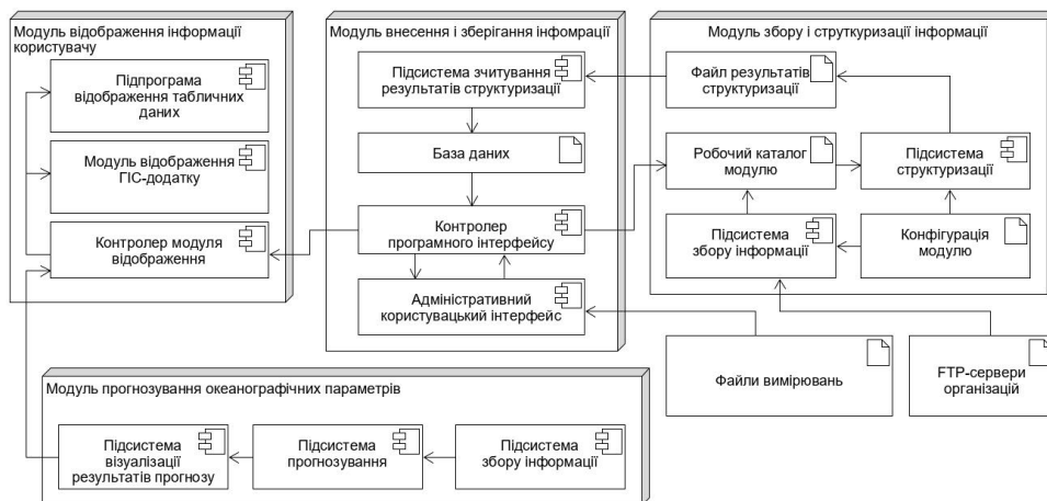
Рис. 1. Архітектура Банку океанографічних даних НАН України
