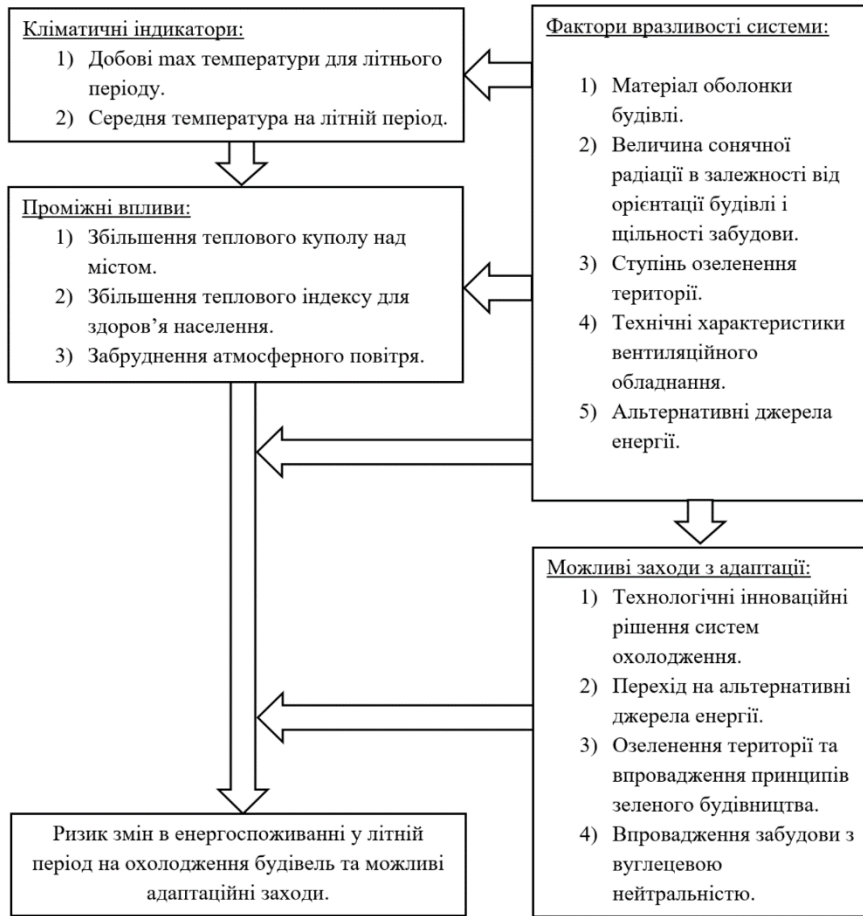
Рис. 1. Ризик змін в енергоспоживанні для будівельного сектору на опалення у зимовий період (А) та на охолодження у літній період (Б) та можливі заходи з адаптації до змін клімату
