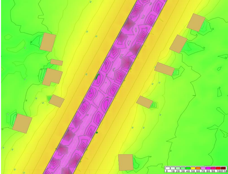
Рисунок 6. Рівні еквівалентного звукового тиску для денного часу L_{A\text{ екв}} , дБА, відмітка +1,500 в н.п. Сепіполки, екран 3 м
