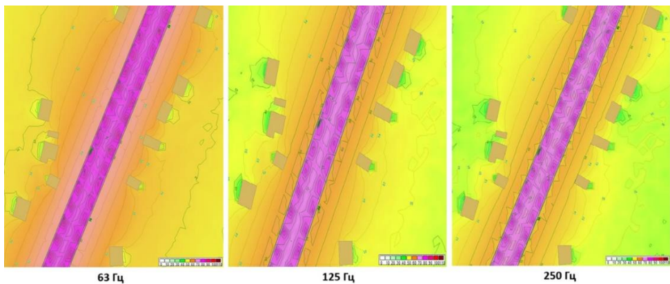
Рисунок 7. Рівні звукового тиску в октавному діапазоні для денного часу, дБ, відмітка +1,500 в н.п. Сепіполки, частоти 63, 125, 250 Гц, екран висотою 3 м
