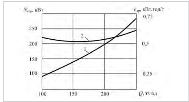
Рис. 2: Зміна потужності, що споживається N_{сep} (1) та питомої енергоємності дроблення e_{др} (2) в залежності від ступеня завантаження дробарки крупного дроблення типу ККД - 1500/180 (Q) Джерело: Власна розробка
