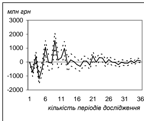
а) відгук ВВП на імпульс M0
