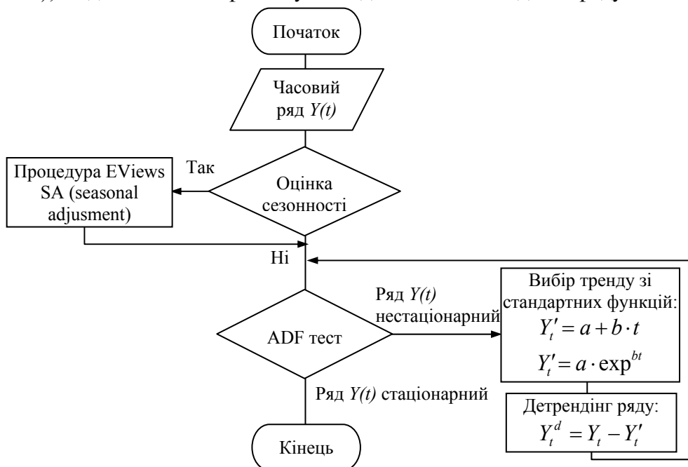
Рис. 2. Алгоритм приведення до стаціонарності методом детрендіngu
