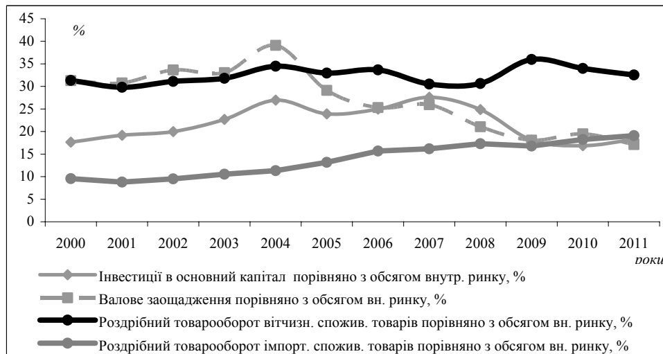
Рис. 2. Динаміка валового заощадження, інвестицій в основний капітал, роздрібного товарообороту вітчизняної та імпоротної продукції на внутрішньому ринку України в 2000–2011 рр.
