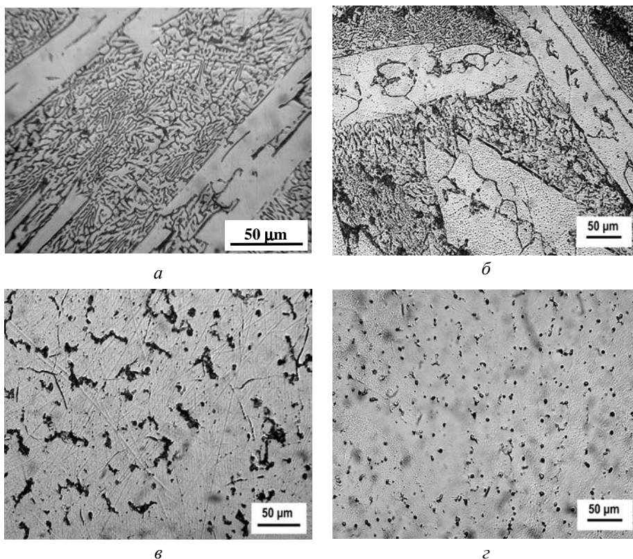
Рис. 1. Микроструктура эвтектического ( L_{12} + \beta )-сплава (№ 1) (а, б) и однофазного L_{12} -интерметаллида (№ 4) (в, з) базовых составов (а, в) и после легирования комплексами элементов (б — сплав № 2, з — сплав № 5).
