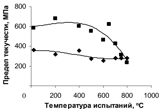
Рис. 2. Температурная зависимость предела текучести сплавов тройной системы Al—Ti—Cr: ♦ — двухфазный эвтектический ( L_{12} + \beta )-сплав (№ 1); ■ — однофазный L_{12} -интерметаллид (№ 4).
