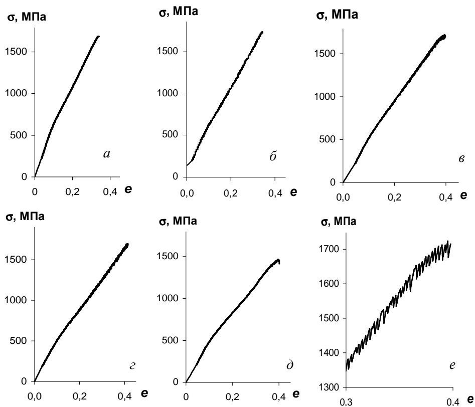
Рис. 3. Диаграммы нагружения в координатах напряжение \sigma — деформация \epsilon эвтектического сплава № 1 при различных температурах испытания ( ^{\circ}\text{C} ): 20 (а), 200 (б), 300 (в), 400 (г), 600 (д); фрагмент диаграммы нагружения при 300 ^{\circ}\text{C} (е).
