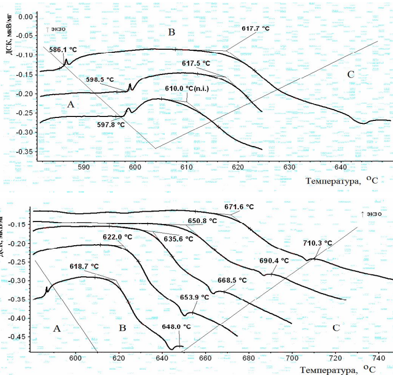
Рис. 2. ДСК кривые плавления сплава Mg—12,5Al—1,4Ca—0,3Y—0,2Gd: a — перефазы 1—3; б — перефазы 4—7.
