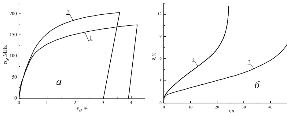
Рис. 8. Кривые деформации при испытаниях на растяжение (а) и длительную прочность (б) сплавов Mg—12,5Al (1) и Mg—12,5Al—0,1Al 3 Zr (2).
