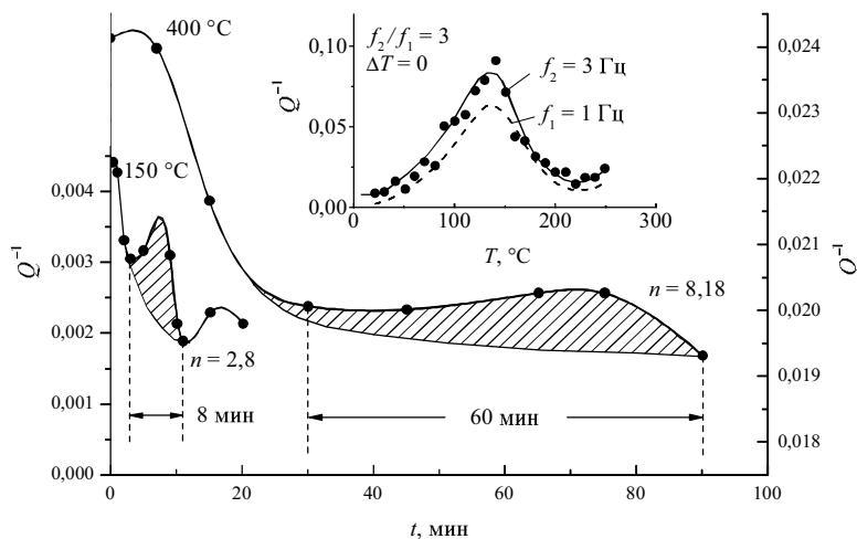
Рис. 4. Кинетические кривые-изотермы амплитудно-независимого внутреннего трения \Delta_{\text{АНВТ}} для сплава Mg—2,1Ba. Вставка: дискретный температурный спектр внутреннего трения Q^{-1} при двух частотах свободного затухания колебаний ( f_1 = 1 и 3 Гц).
