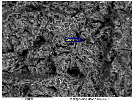
Рис. 7. Микрофотография РЭМ поверхности разрушения сплава Mg—12,5Al—1,4Ca—0,3Mn, модифицированного добавками 0,2Ti с локальным химическим составом \alpha -Mg и \beta -Mg 17 Al 12 (x).
