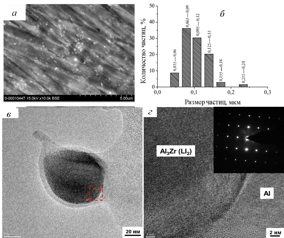
Рис. 1. Микрофотография РЭМ нанодискретной лигатуры (а) и диаграмма распределения интерметаллидных частиц \text{Al}_3\text{Zr} по размерам (б); картина электронной микродифракции интерметаллидных частиц \text{Al}_3\text{Zr} с кубической решеткой типа \text{L1}_2 и с изображениями выбранных участков высокого разрешения (в, з).
