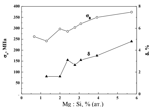
Рис. 4. Механические свойства нелегированных сплавов вдоль линии моновариантного эвтектического превращения L \rightleftharpoons \alpha\text{-Al} + Mg_2Si .
