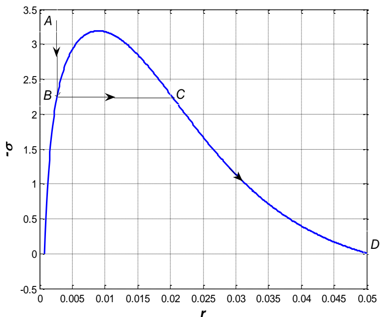
Рис. 2. Трехстадийный процесс эволюции трещины с размером r < 0.01 м. Этап АВ – адиабатическое увеличение зияния трещины, этап ВС – резкое увеличение радиуса, этап 3 – плавный рост объема трещины в целом. Кривая страгивания отвечает быстрой разгрузке угольного пласта, т.е. адиабатическому расширению газа внутри полости трещины ( \kappa = 4/3 ). Предполагается, что полость трещины заполнена метаном
