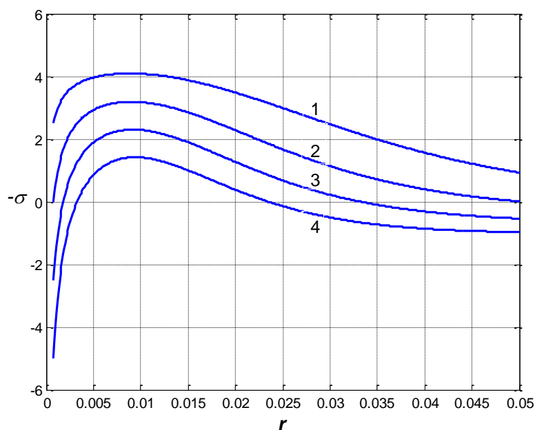
Рис. 4. Кривые страгивания в зависимости от модуля сцепления угля K . Кривые 1 – 4 отвечают значениям модулей сцепления K_1 = 10^5 \text{H}/\text{m}^{3/2} ; K_2 = 2 \cdot 10^5 \text{H}/\text{m}^{3/2} ; K_3 = 3 \cdot 10^5 \text{H}/\text{m}^{3/2} ; K_4 = 4 \cdot 10^5 \text{H}/\text{m}^{3/2} соответственно. По осям \sigma - критическое внешнее напряжение страгивания; r - радиус трещины. Процесс сброса внешнего напряжения предполагается быстрым (адиабатическим)
