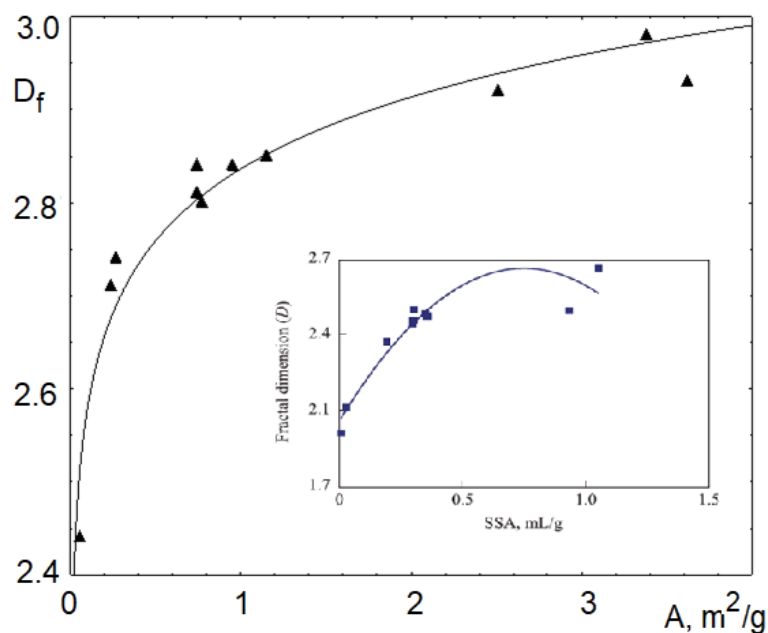
Рис. 2. Связь поверхностной фрактальной размерности с удельной поверхностью углей по данным МУРН. На врезке для сравнения приводится рисунок из статьи [20]
