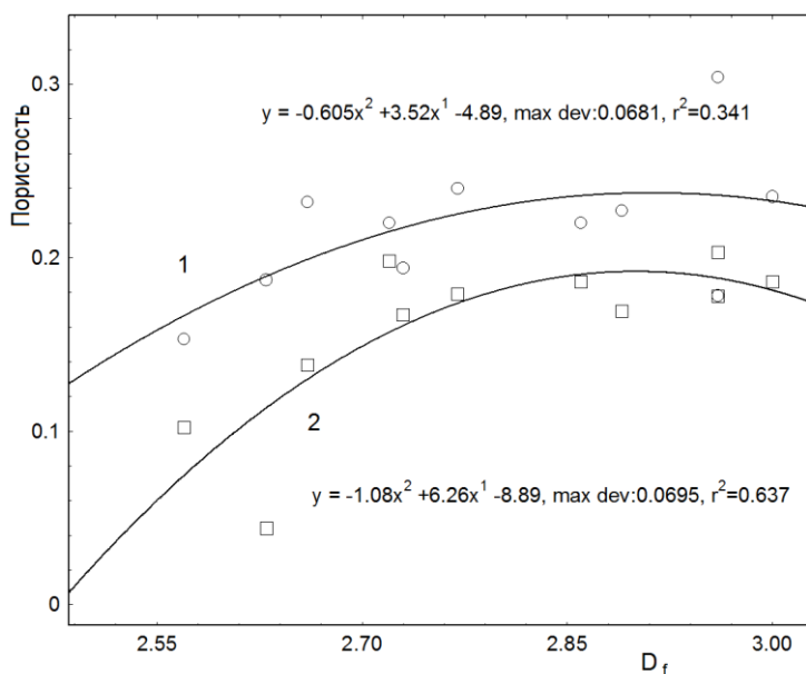
Рис. 4. Зависимость пористости углей от фрактальной размерности: 1 - полная, 2 - закрытая пористость
