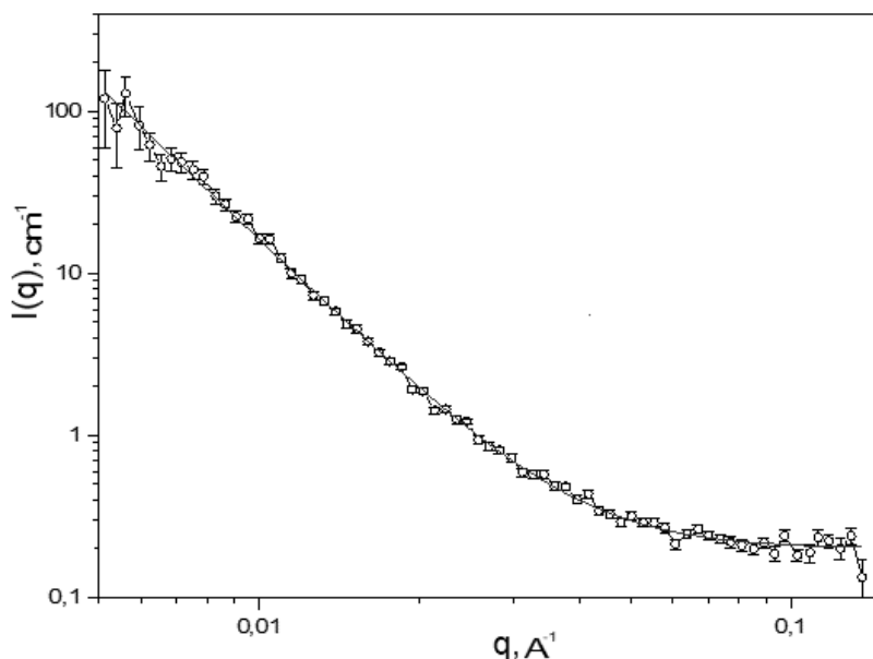
Рис. 1. Экспериментальная кривая рассеяния нейтронов для образца угля марки Т (ГП «Макеевуголь» ш. им. С.М. Кирова, пласт H^B_{10} ), построенная в двойных логарифмически координатах
