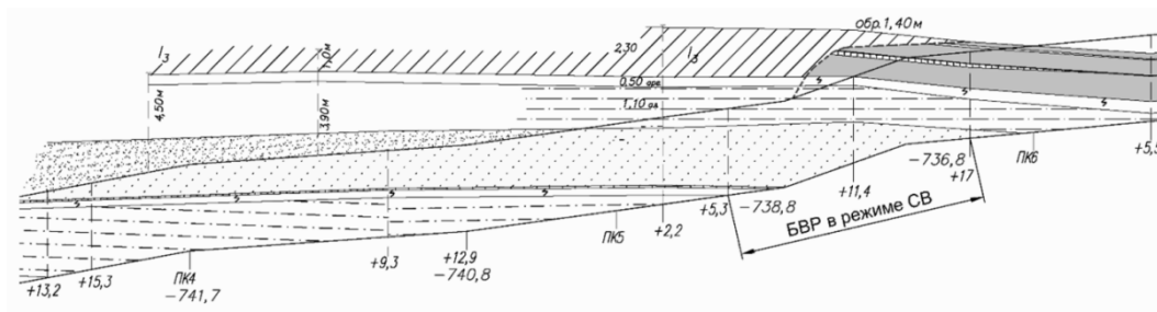
Рис. 1. Геологический разрез по трассе вскрывающей выработки угольный пласт l_3
