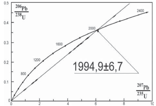
Рис. 7. Уран-свинцева діаграма з конкордією для уламків кристалів уранового мінералу із плагіопегматиту, пр. 23/23
