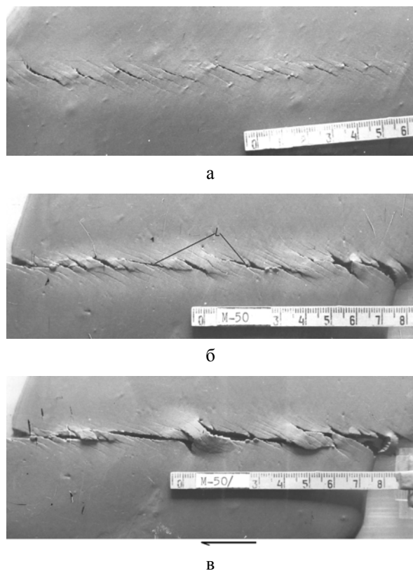
Рис. 8. Тристадійний розвиток ЗГЗ в моделі з кварцового піску та гліцерину (пояснення в тексті)
