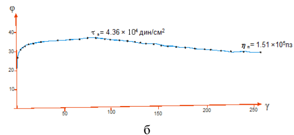
Рис. 6. Реологічні криві для паст на основі кварцового піску (концентрація 84,6 %) та технічного гліцерину: а – фракція піску з розмірами зерен 0,05–0,63 мм; б – з розмірами зерен \leq 0,05 мм
