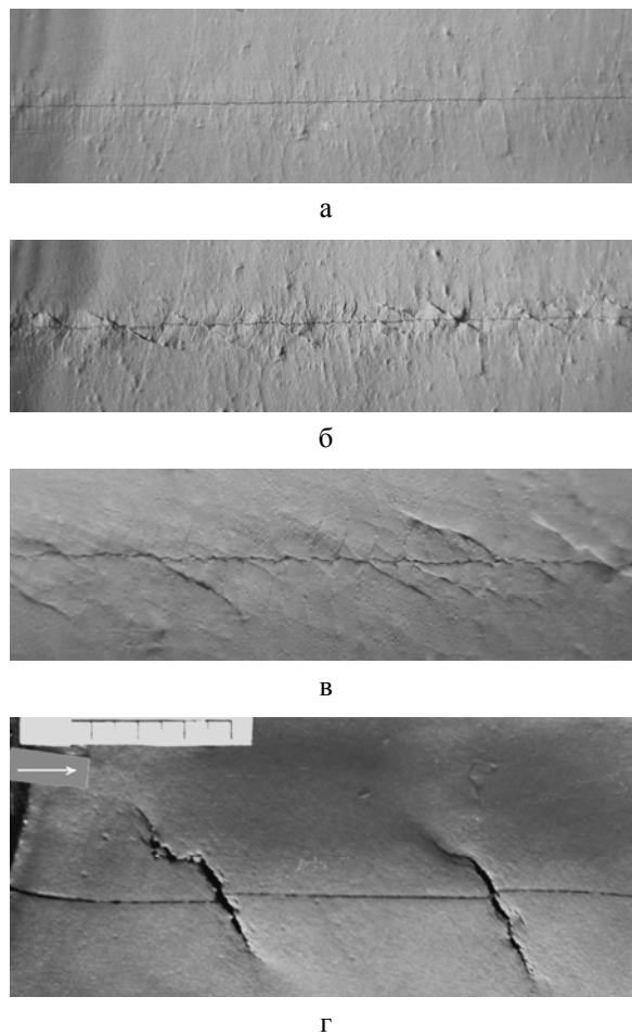
Рис. 9. Розвиток ЗГЗ у моделях з кварцового піску та вазелінової олії (фракція піску з розмірами зерен 0,05–0,63 мм, концентрація 80,8 %)
