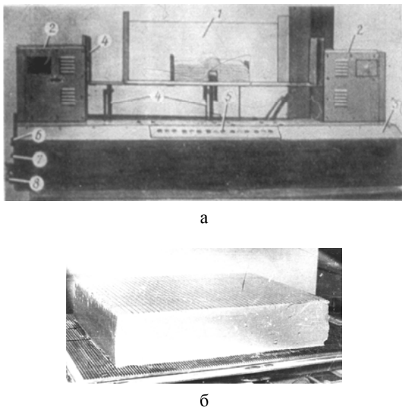
Рис. 1. Установа фізичного моделювання процесів розривотворення на пластично-в'язких матеріалах (а) та модель з глинистої пасти (б)
