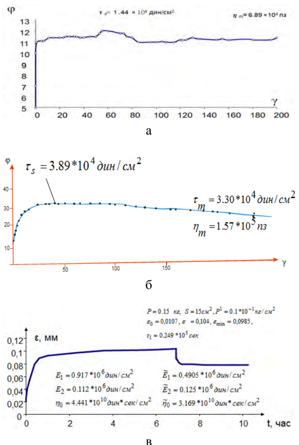
Рис. 2. Реологічні властивості глинистих паст: а – реологічна крива \tau(\varepsilon) при \varepsilon = \text{const} для глинистої пасти; б – те ж для пасти аеросил (15 %) – вазелінова олія (85 %); в – крива кінетики деформації для пасти Веселовської глини (концентрація 58,6 %)
