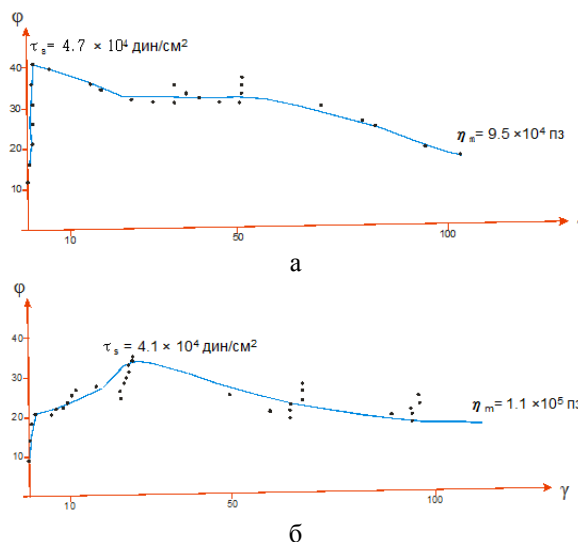
Рис. 10. Реологічні криві для паст на основі піску та вазелінової олії: а – фракція піску з розмірами зерен 0,05–0,63 мм (концентрація 82,14 %); б – з розмірами зерен \leq 0,05 мм (концентрація 79,38 %)
