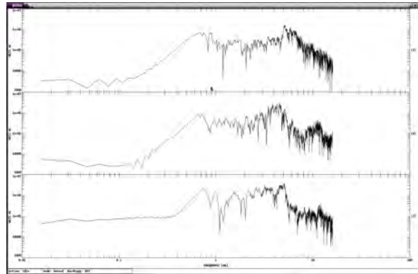
Рис. 3. Спектральні характеристики сейсмічних сигналів по трьох компонентах Z, N, E землетрус у Кривому Розі 23.06.2013
