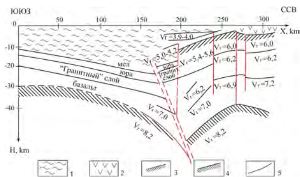
Рис. 1. Профиль ГСЗ по линии Огурчинский-Сарыкамыш
