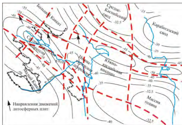
Рис. 2. Схема тектоники ЮКМ и смежных территорий по подошве земной коры
