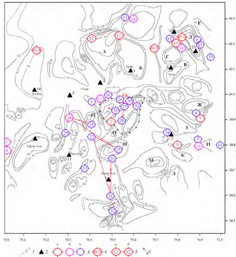
Рис. 1. Пространственное распределение эпицентров сильных землетрясений Гармского района. 1 – глубина кровли слоя сильного поглощения в км; 2 – сейсмические станции; 3 – эпицентры землетрясений с M > 6, 5.5, 5.0 ; 4 – положение эпицентров землетрясений по палеосейсмодислокациям, 5 – эпицентры Гармского 1941 г. землетрясения по разным источникам; 6 – границы конгломерата блоков Каудальской зоны (стрелками показана последовательность его деконсолидации). Цифры – номера землетрясений, которые произошли соответственно: 13.11.1895(1), 16.9.1924(2), 2.1.1925(3), 30.6.1926(4), 31.8.1934(5), 3.9.1934(6), 11.9.1934(7), 4.1.1935(8), 8.10.1935(9), 12.1.1938(10), 30.5.1939(11), 20.4.1941(12), 26.4.1941(13), 6.5.1941(14), 28.2.1942(15), 28.5.1942(16), 8.7.1949 (7 ч 50 мин.) (17), 8.7.1949 (8 ч 02 мин.) (18), 10.7.1949(19), 17.11.1950(20), 21.11.1950(21), 11.4.1956(22), 13.1.1957(23), 7.1.1958(24), 31.7.1959(25), 11.4.1966(26), 14.4.1966(27), 22.3.1969(28), 9.6.1975(29), 3.9.1976(30), 25.12.1977(31), 17.11.1978(32), 26.2.1983(33), 21.12.1987(34), 20.2.1995(35), 21.7.2007(36), 13.10.2008(37) ( http://seismorus.ru/eq_cat ).
