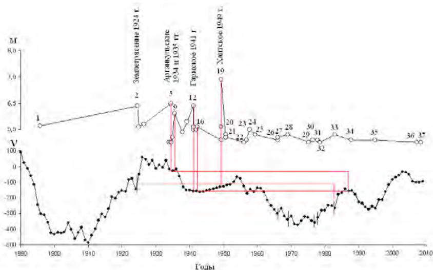
Рис. 2. Вариации скорости вращения Земли и сильные землетрясения с M > 5.0 . Гармского района из каталога http://seismorus.ru/eq_cat . Цифры соответствуют рис.1. Рисками отмечены землетрясения, локализованные в Каудальской зоне.
