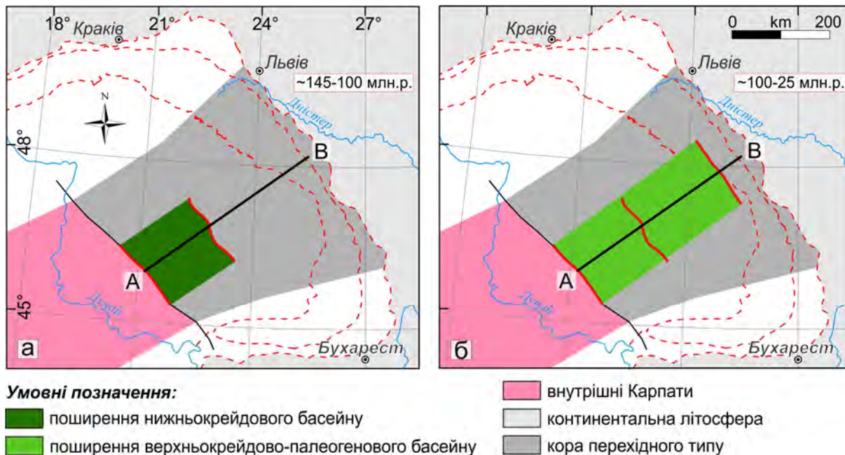
Рис. 8. Палеогеографічна карта Східних Карпат на крейдово-палеогеновий час
