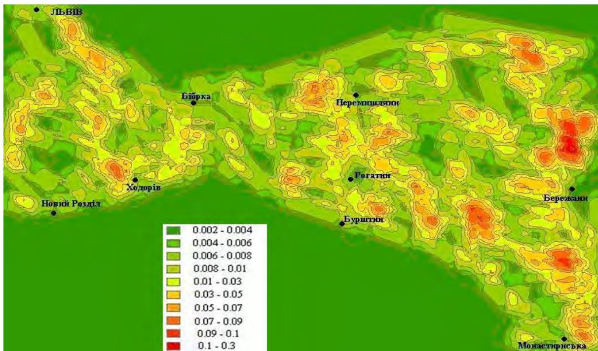
Рис. 6. Щільність лінеаментів різних рангів у межах височини Опілля, км/км 2 (масштаб 1:200 000) Fig. 6. The density of lineaments different ranks within height Opilla in km/км 2 (scale 1: 200 000)
