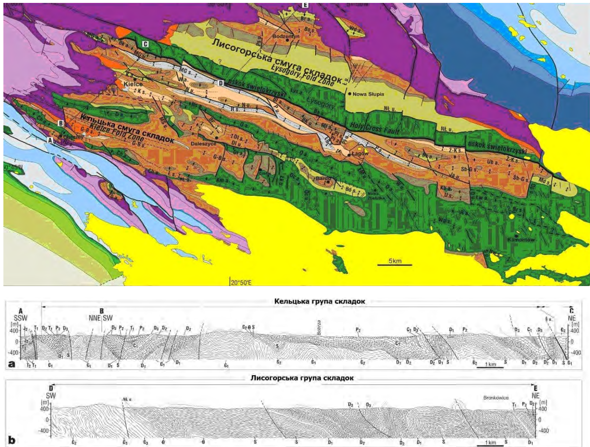
Рис. 2. Геологічна карта і профіль через кельцьку і лисогорську групи складок Свентокшицьких гір (А. Konon, 2008)
