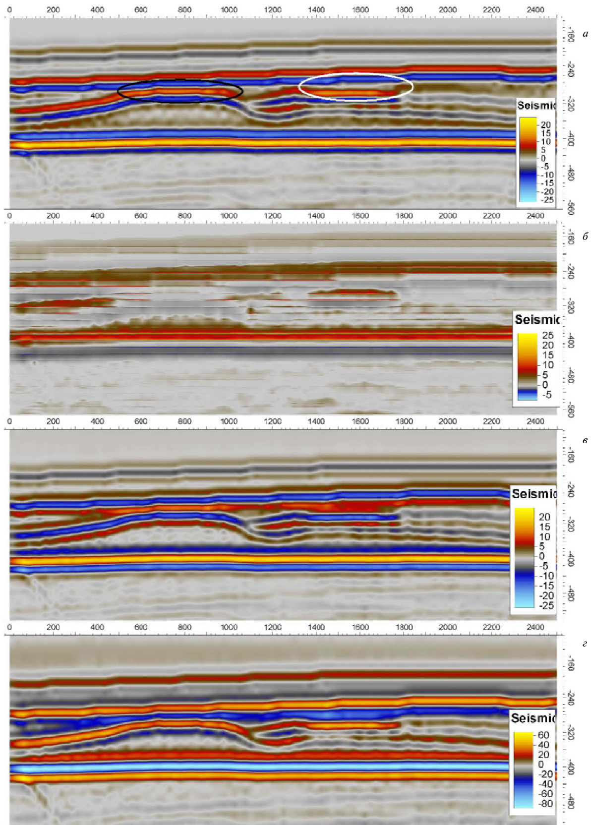
Рис. 3. Сейсмічний розріз геологічної моделі (а), комплекс вибраних “диференційних” сейсмічних атрибутів – перша похідна миттєвої амплітуди (б), квадратура амплітуди (е), відносний акустичний імпеданс (з). Білим виділено зону колектору, чорним – зону інтерференції
