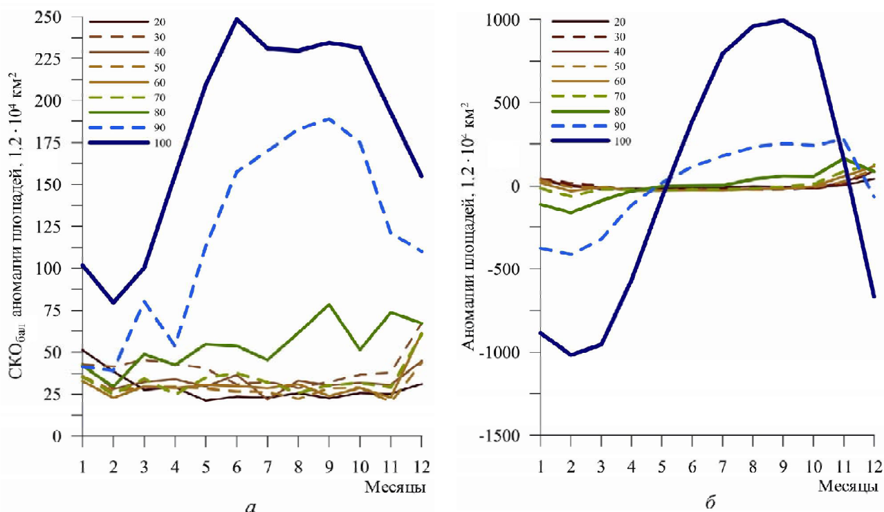
Рис. 2. Изменение по месяцам межгодовых среднеквадратических отклонений (а) и климатический сезонный цикл (б) аномалий площадей морских льдов разной балльности (ед. 1,2 \cdot 10^4 \text{ км}^2 )
