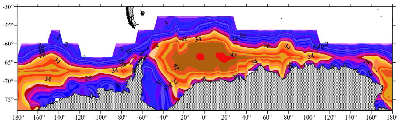
Рис. 1. Распределение SKO_{сез} (%) морских льдов Антарктики
